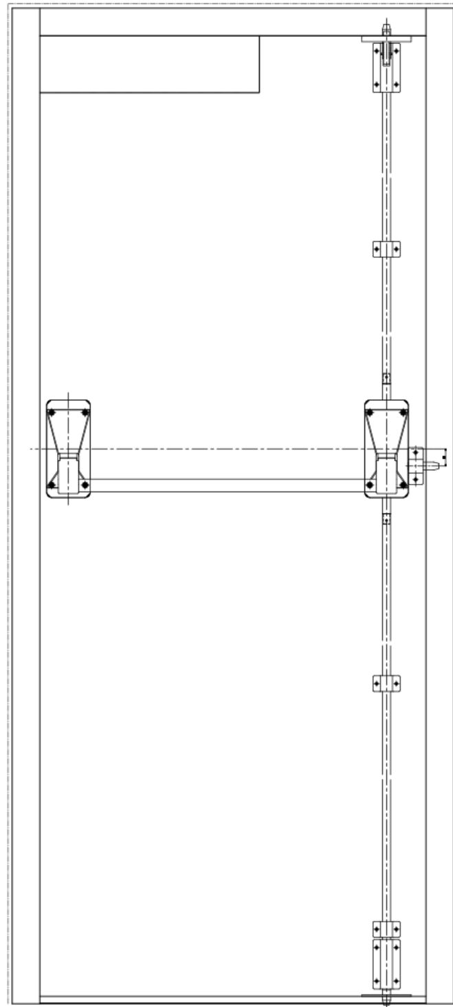
1 ELEVATION SCALE 1:1
